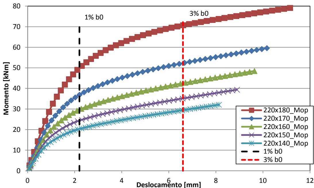
Figura 43 – Curva momento versus deslocamento ( M_{op} ) – SHS 220x220x8.
