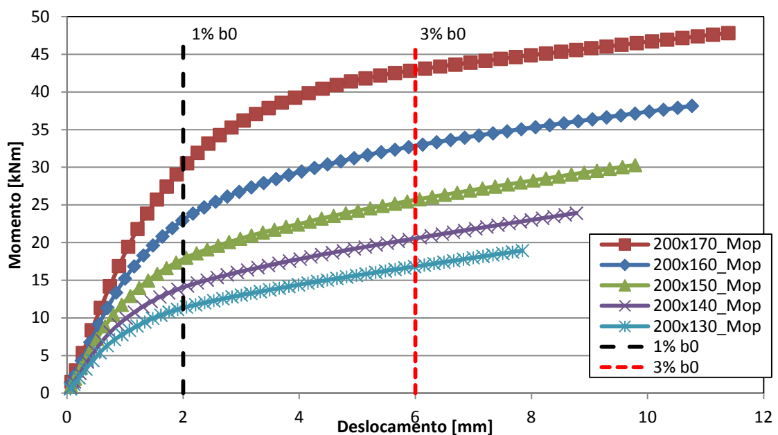
Figura 42 – Curva momento versus deslocamento ( M_{op} ) – SHS 200x200x6.
