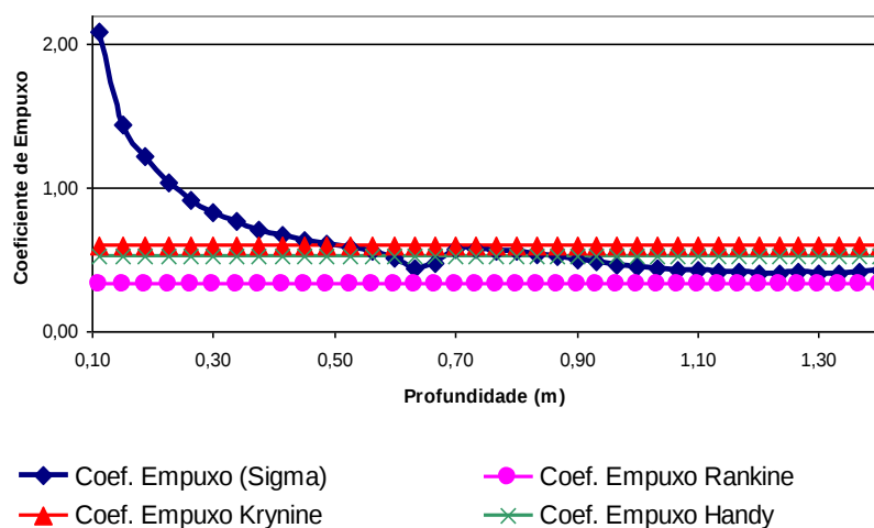
Figura 36 – Comparação entre coeficientes de empuxo ( H = 0,90\text{m} ). (Ferreira, 2007)
