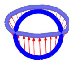
Figura 96 – Elevação localizada - Deflexões do duto na seção S1 para \delta/B = 2\% (sem elemento de interface).
