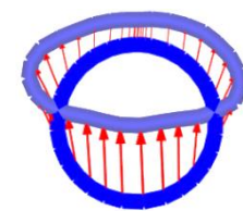
Figura 97 – Elevação localizada - Deflexões do duto na seção S1 para \delta/B = 4\% (sem elemento de interface)
