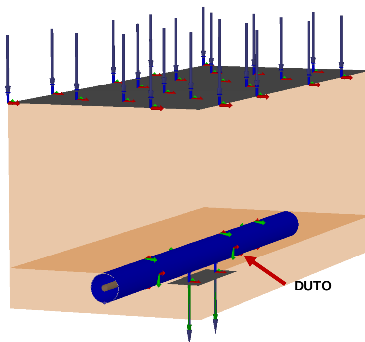
Figura 57 – Modelo de tubo de PVC: elemento de placa.
