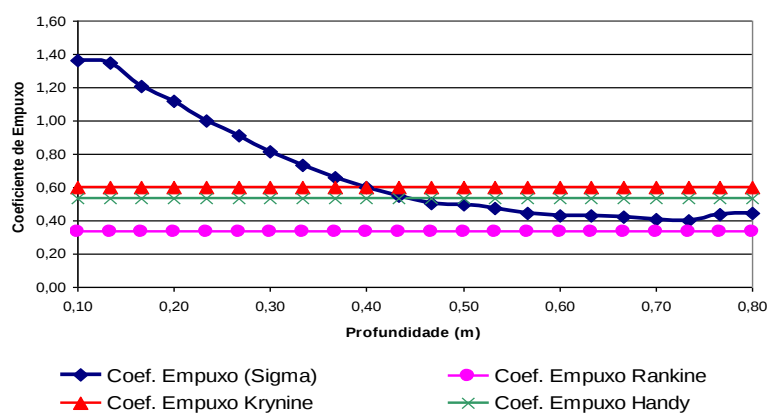
Figura 34 – Comparação entre coeficientes de empuxo ( H = 0,30\text{m} ). (Ferreira, 2007)
