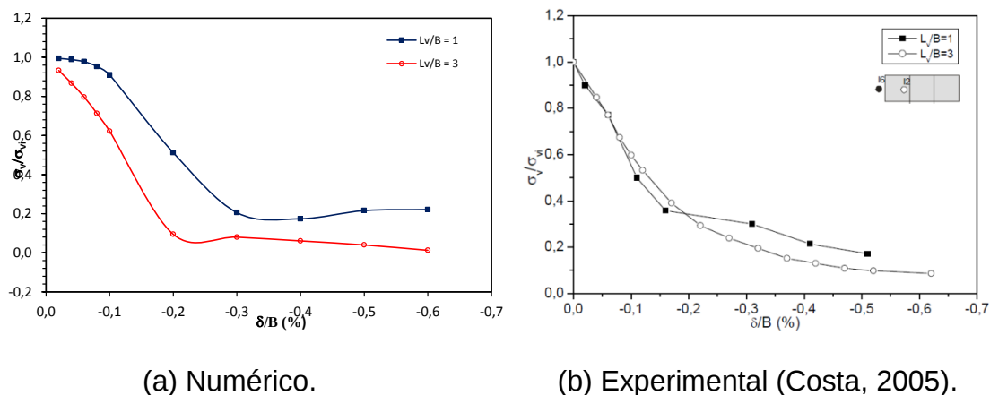
Figura 76 – Comportamento da tensão vertical no exterior do alçapão retangular e do quadrado, na longitudinal, em arqueamento passivo; D_r = 100\% e q = 100 kPa.
