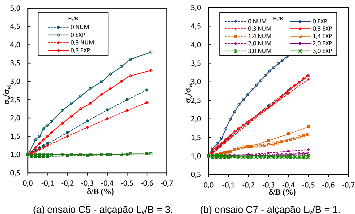
Figura 73 – Variação da tensão vertical em um perfil vertical no centro do alçapão; D_r = 100\% e q = 100 \text{ kPa} .
