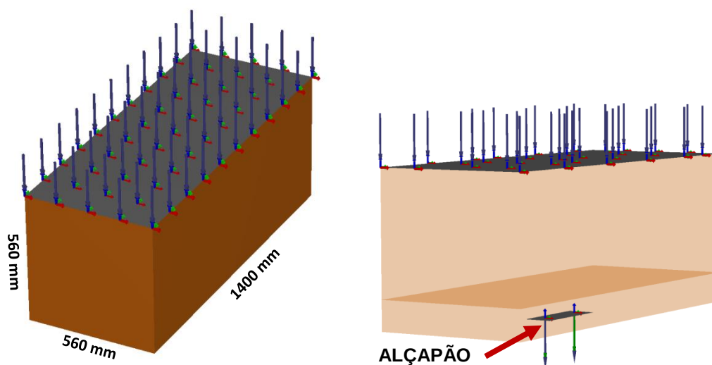
Figura 56 – Geometria dos ensaios de arqueamento, série C.
