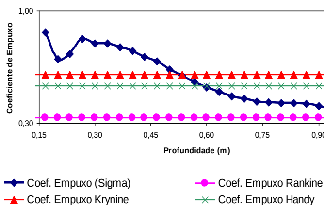
Figura 35 – Comparação entre coeficientes de empuxo ( H = 0,50\text{m} ). (Ferreira, 2007)
