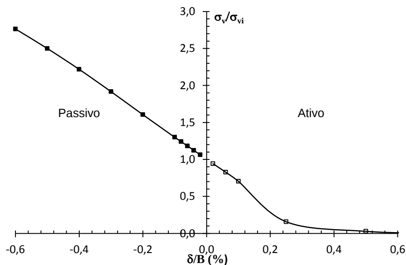
Figura 77 – Variação da tensão no centro do alçapão com o deslocamento em arqueamento ativo e passivo. D_r = 100\% e q = 100 kPa.
