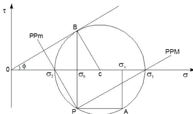
Figura 18 – Círculo de Mohr descrito por Krynine (1945) para determinação do coeficiente de empuxo.
