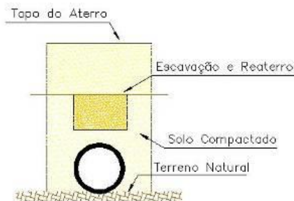
Figura 14 – Conduto em Condição de Pseudovala.
