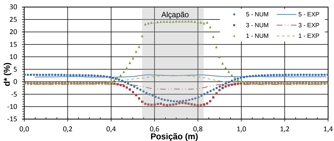
Figura 96 – Elevação localizada - Deflexões do duto na seção S1 para \delta/B = 2\% (sem elemento de interface).
