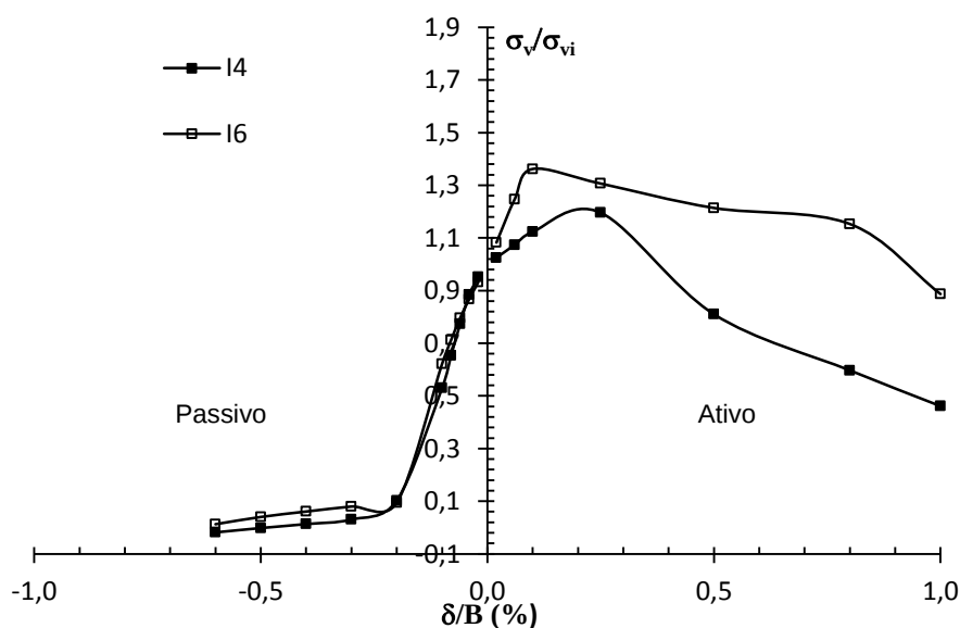
Figura 78 – Variação da tensão no exterior do alçapão com o deslocamento em arqueamento ativo e passivo. D_r = 100\% e q = 100 kPa.
