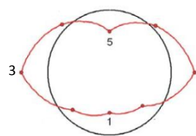
Figura 97 – Elevação localizada - Deflexões do duto na seção S1 para \delta/B = 4\% (sem elemento de interface)
