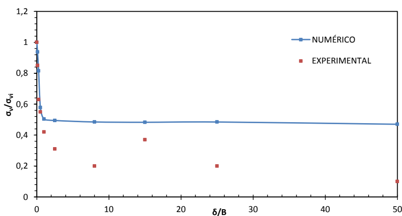
Figura 79 – Variação da tensão vertical no topo do duto ao longo da translação do alçapão, no modelo MC. Ensaio D7 (perda de apoio).
