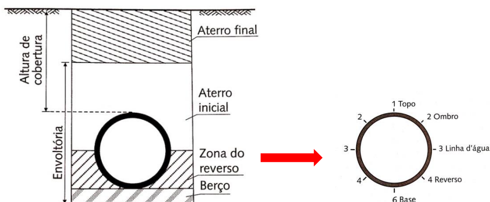
Figura 10 – Definição dos elementos constituintes de uma instalação típica e identificação dos locais da seção transversal do duto, (Bueno e Costa, 2012).
