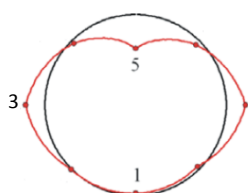
Figura 96 – Elevação localizada - Deflexões do duto na seção S1 para \delta/B = 2\% (sem elemento de interface).
