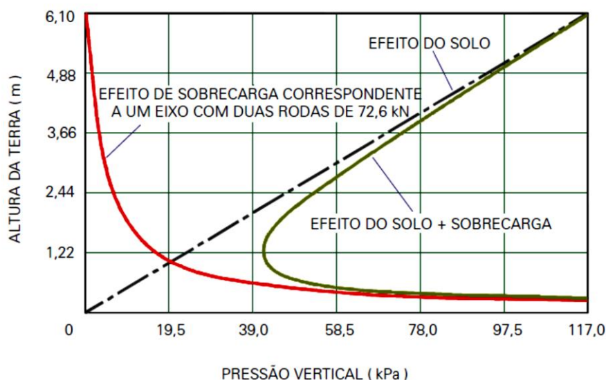
Figura 24 – Pressão vertical versus altura de embutimento em plano horizontal sobre o duto para trem-tipo H-20: 2 rodas, pesando 72,6kN e área de contato de 45,7cm x 50,8cm, distantes entre si de 1,83m (Debs, 2003).
