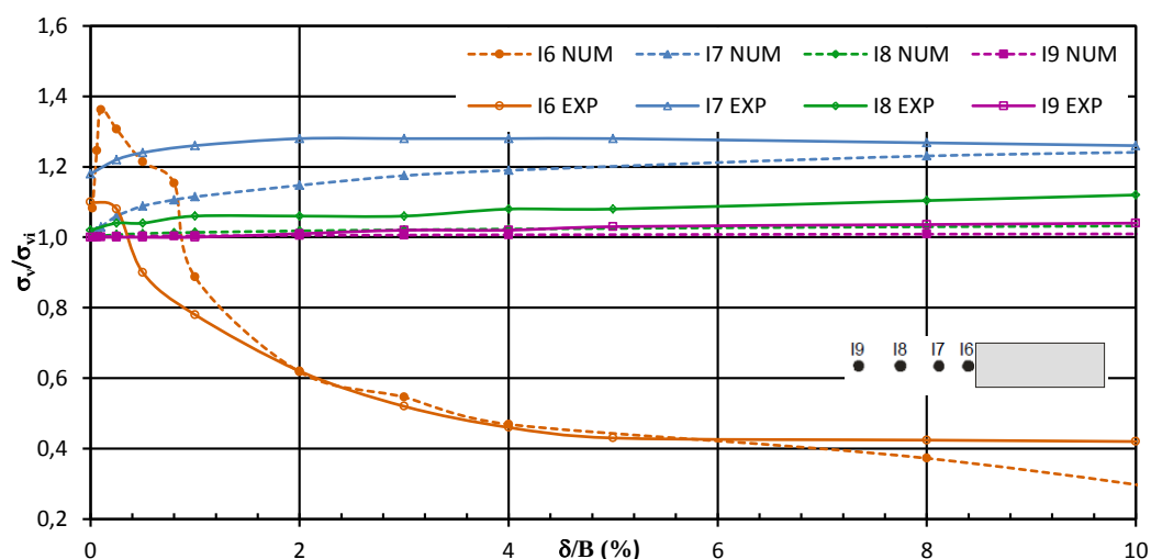
Figura 63 – Variação da tensão vertical no exterior do alçapão na direção longitudinal– Ensaio C2 D_r = 100\% e q = 100 kPa alçapão L_v/B = 3 .
