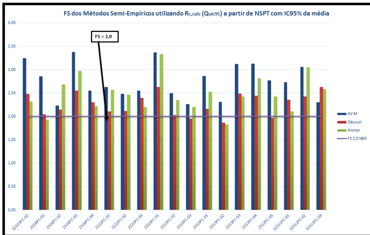
Figura 54 – Gráfico de barras onde se pode observar os FSg por método de estimativa de capacidade de carga, por estaca e por região.
