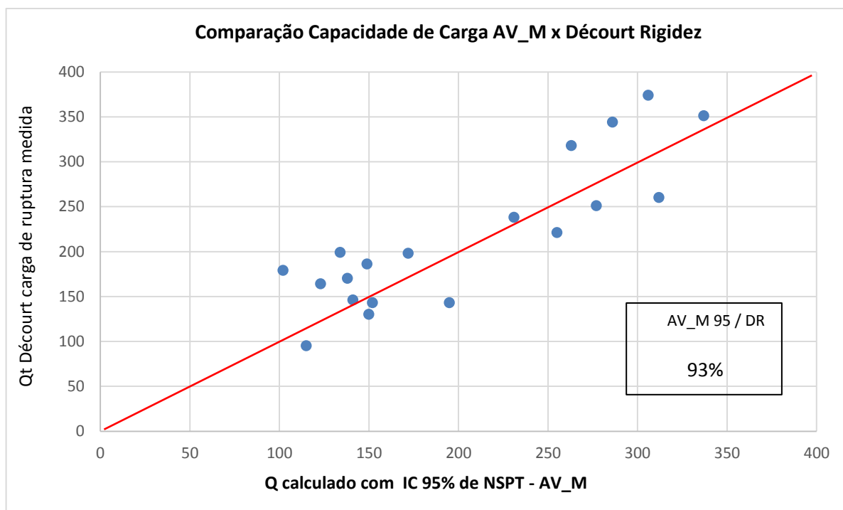
Figura 49 - Carga de ruptura extrapolada por Décourt (Rigidez) versus a capacidade de carga de estimada com N_{SPT} 95% MED, para Aoki-Velloso.
