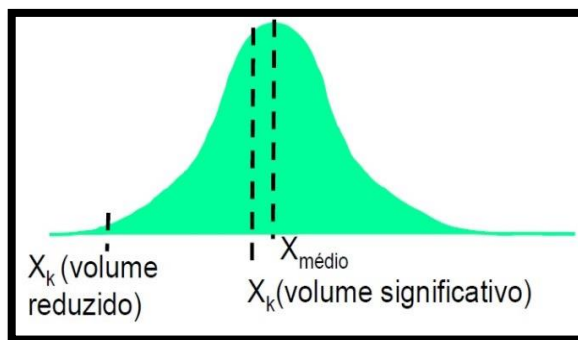
Figura 24 – Distribuição do parâmetro de resistência de um terreno (Alves, 2013).
