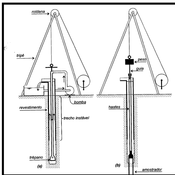
Figura 7 – Etapas na execução de sondagem a percussão: a) avanço da sondagem por desagregação e lavagem e b) ensaio de penetração dinâmica. (Velloso e Lopes, 1996).
