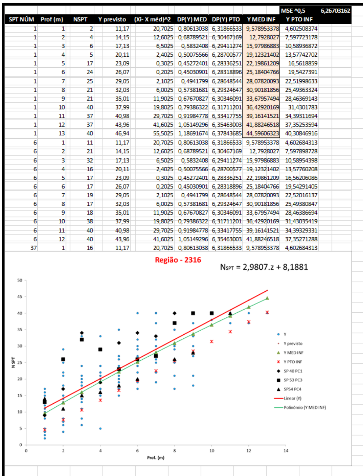
Figura 37 – Cálculos e Gráfico com a curva inferior na cor verde ( Y_{\text{MED INF}} ) dos valores de N_{\text{SPT}} obtidos conforme aplicação do critério estatístico.
