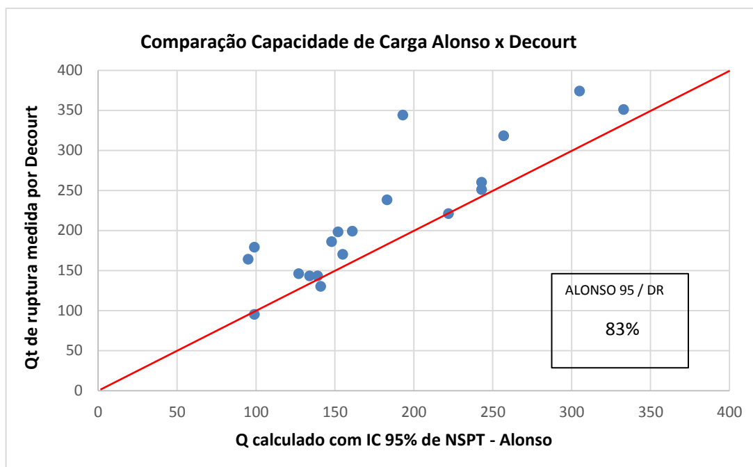
Figura 53 - Carga de ruptura extrapolada por Décourt (Rigidez) versus a capacidade de carga estimada com N_{SPT} 95% MED, para Alonso.
