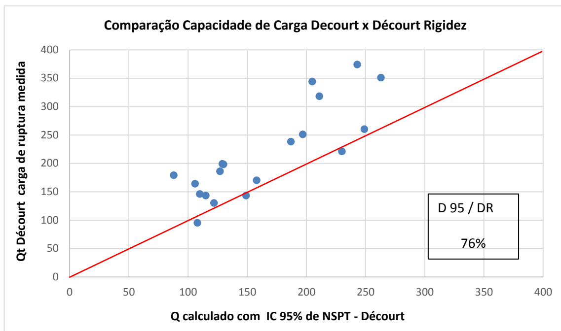
Figura 51 - Carga de ruptura extrapolada por Décourt (Rigidez) versus a capacidade de carga estimada com N_{SPT} 95% MED, para Décourt & Quaresma.
