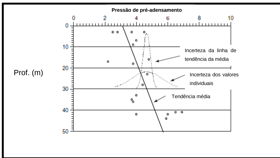
Figura 22 – Distribuições preditivas das pressões máximas médias e pontuais de pré-adensamento, a 30 metros de profundidade (adaptado de Baecher e Christian, 2003).
