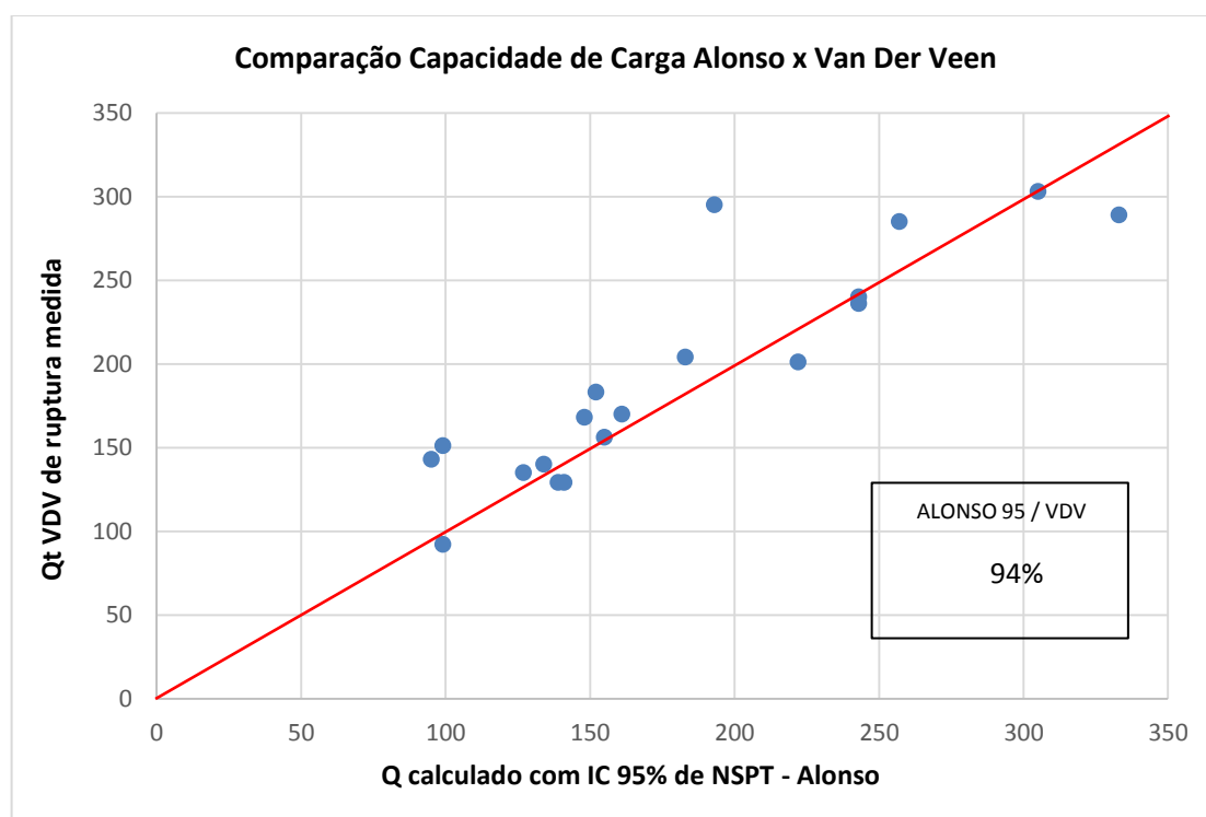
Figura 52 - Carga de ruptura extrapolada por Van Der Veen versus a capacidade de carga estimada com N_{SPT} 95% MED, para Alonso.
