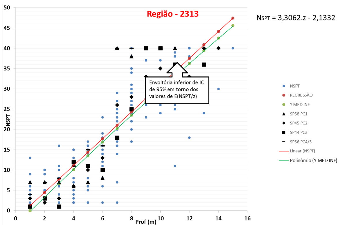
Figura 42 - Envoltória inferior de valores de N_{SPT} em profundidade, região 2313, conforme critério estatístico aplicado.
