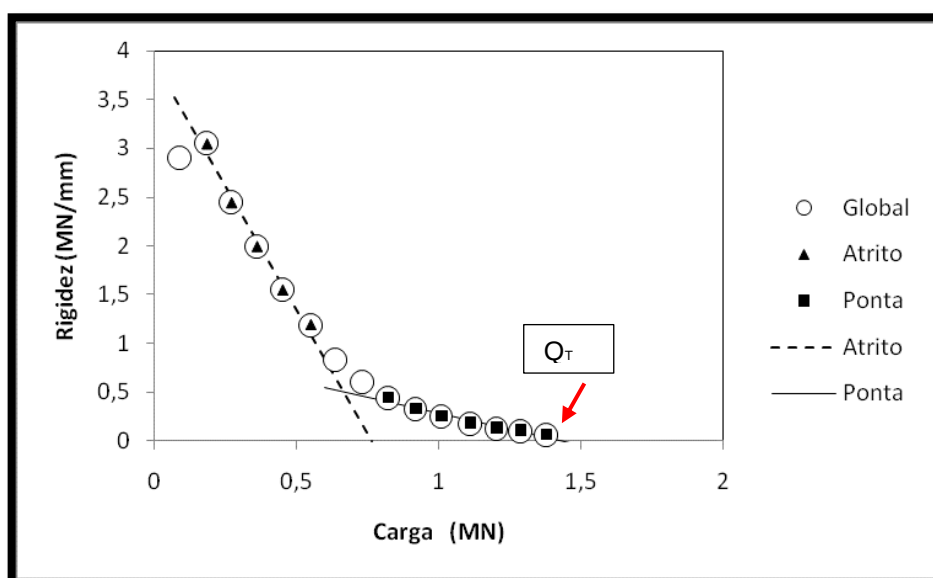
Figura 30 – Método de Décourt, 1996 (adaptado de Pacheco, 2008)
