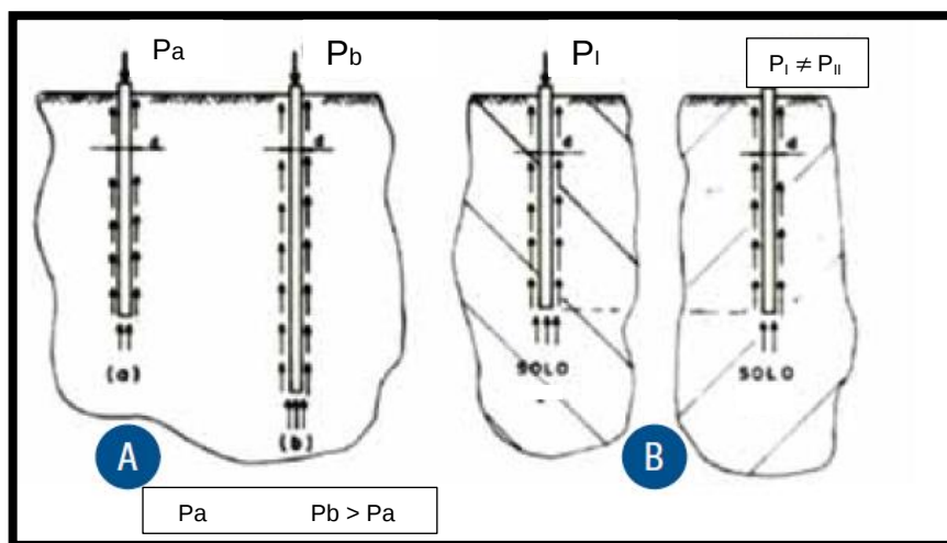
Figura 28 – Estacas e cargas admissíveis (Alonso, 2012).
