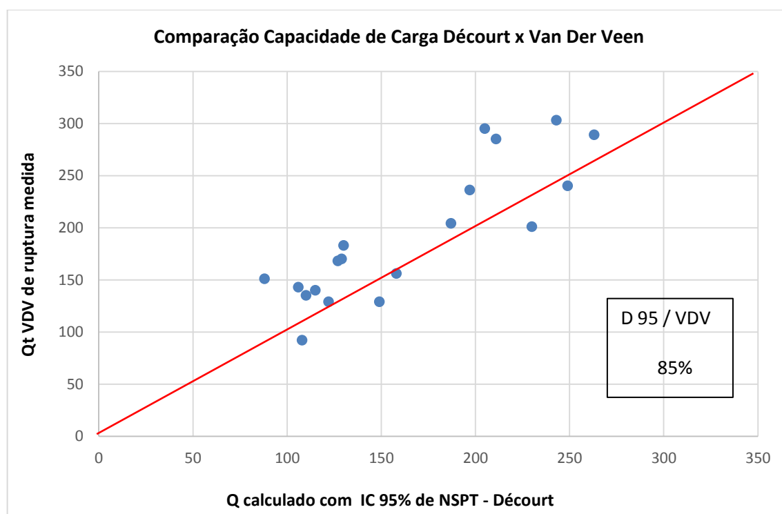
Figura 50 - Carga de ruptura extrapolada por Van Der Veen versus a capacidade de carga estimada com N_{SPT} 95% MED, para Décourt & Quaresma.
