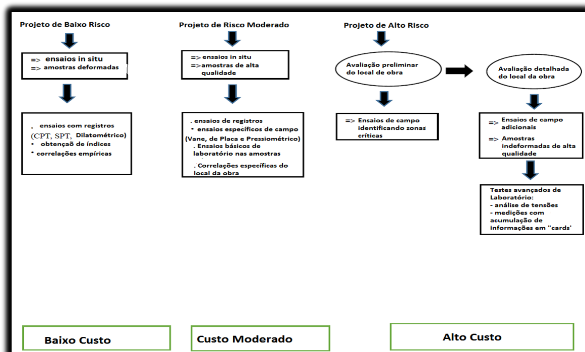
Figura 1 – Investigação do solo baseada em risco (adaptado de Lacasse e Nadim, 1998)
