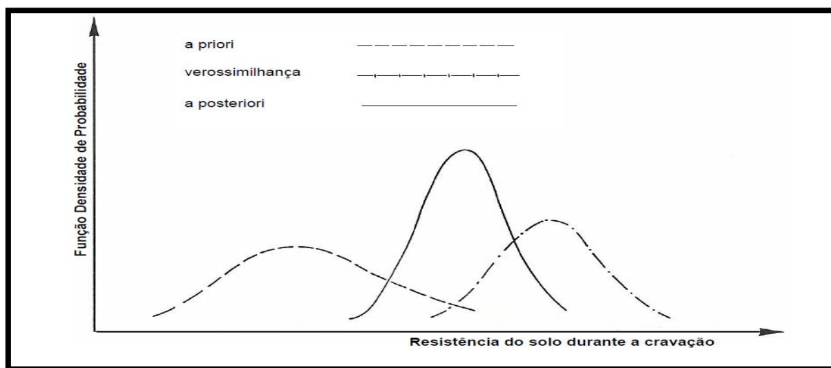
Figura 14 – Correção de distribuições de resistência do solo durante a cravação da estaca (Cabral, 2008).
