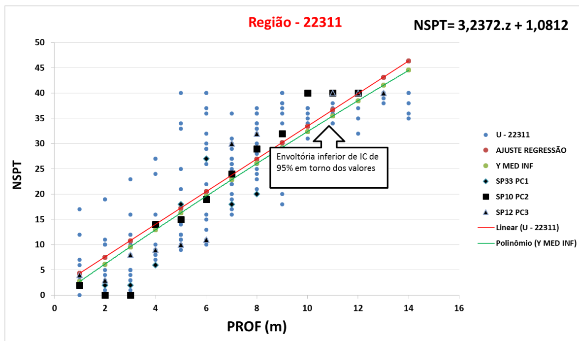
Figura 43 - Envoltória inferior de valores de N_{SPT} em profundidade, região 22311, conforme critério estatístico aplicado
